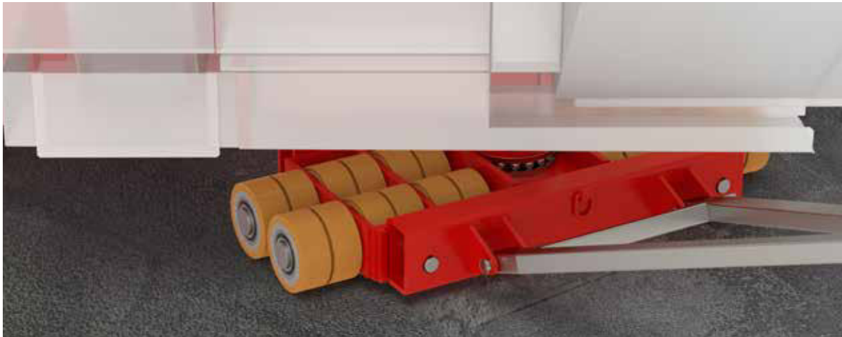
Lenkwerk der H-Serie im Einsatz
